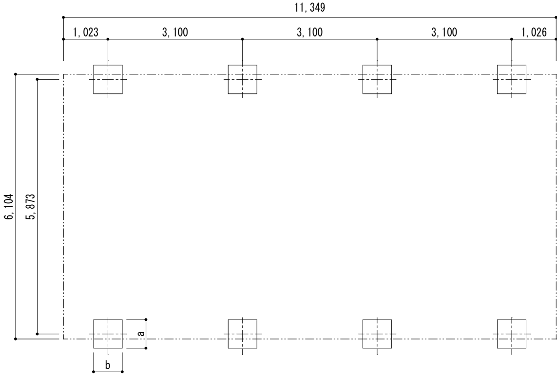
■基礎配置図
